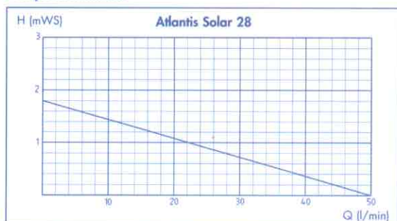
Pumpenkennlinien
